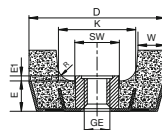
形状 6ZT (インサートナット突出あり)
