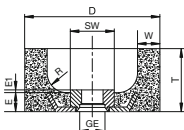
形状 6ZB (挿入ナット突出あり)
