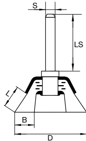
Abmessungen Topfschaftbürsten
