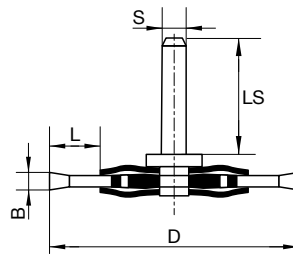
Abmessungen Rundschaftbürsten
