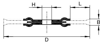
Abmessungen Rundbürsten
